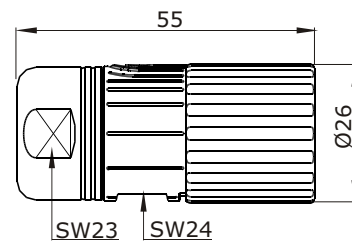
Hauptabmessungen Stecker
