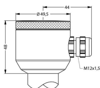
Kompakt-Feldgehäuse (IP 67)
