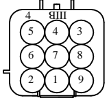
DJK7091-2.3-11 9Pin公头接插件（从入线端看）
