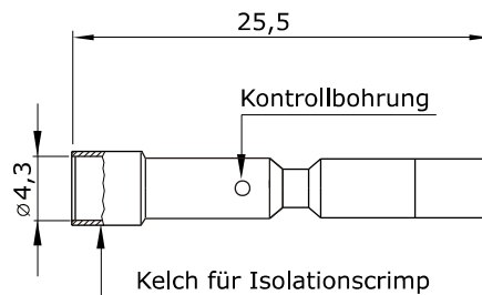
Hauptabmessungen Kontaktbuchse
