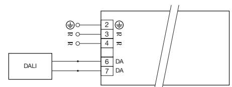
DALI PCA T5 ECO Ip xtec II
